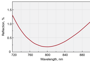
R&lt;0.5% @ 760-840 nm, AOI= 0°
